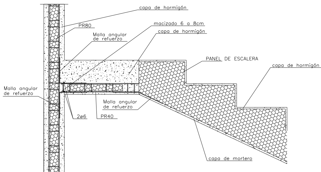
SECCION POR POLIESTIRENO
